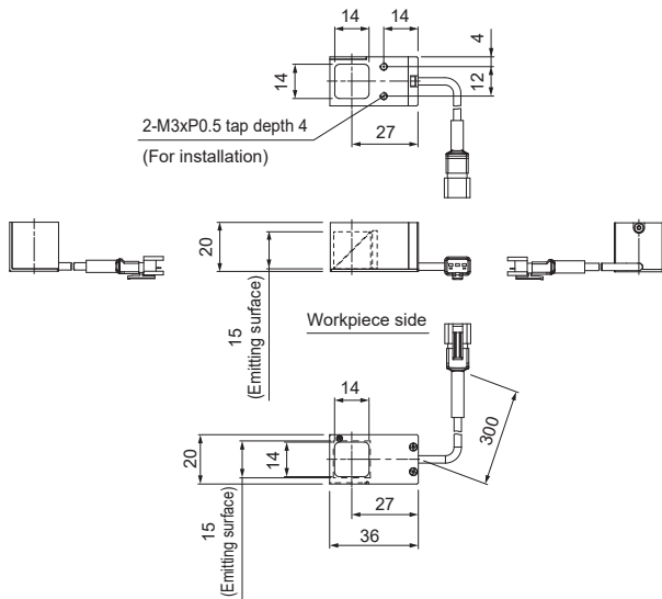
LFV3-CP-13RD/SW/BL
