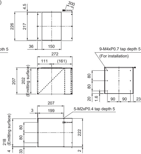
LFV3-200RD(A)/SW(A)/BL(A)
