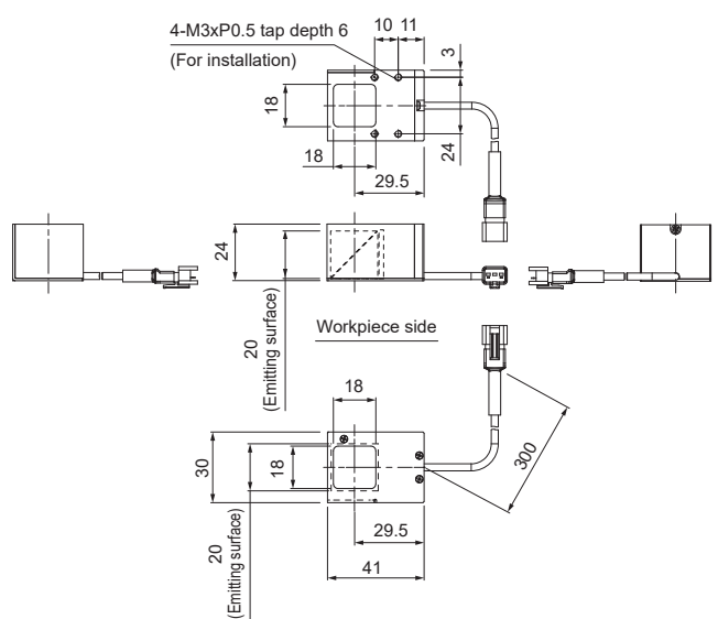
LFV3-CP-18RD/SW/BL
