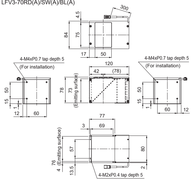
LFV3-70RD(A)/SW(A)/BL(A)
